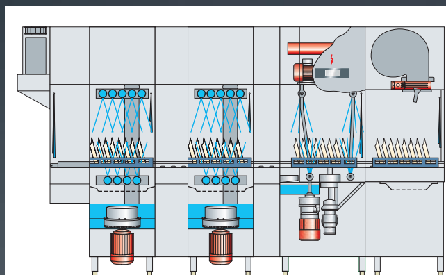
Průřez myčkou UPster® K-M 280
