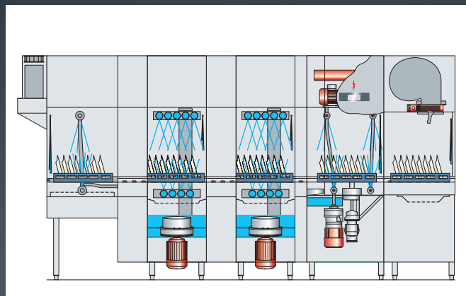
Průřez myčkou UPster® K-L 340
