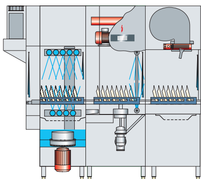
Průřez myčkou UPster® K-S 160
