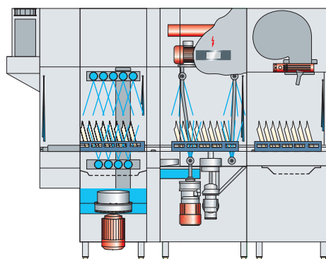
Průřez myčkou UPster® K-S 200
