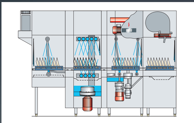
Průřez myčkou UPster® K-M 250
